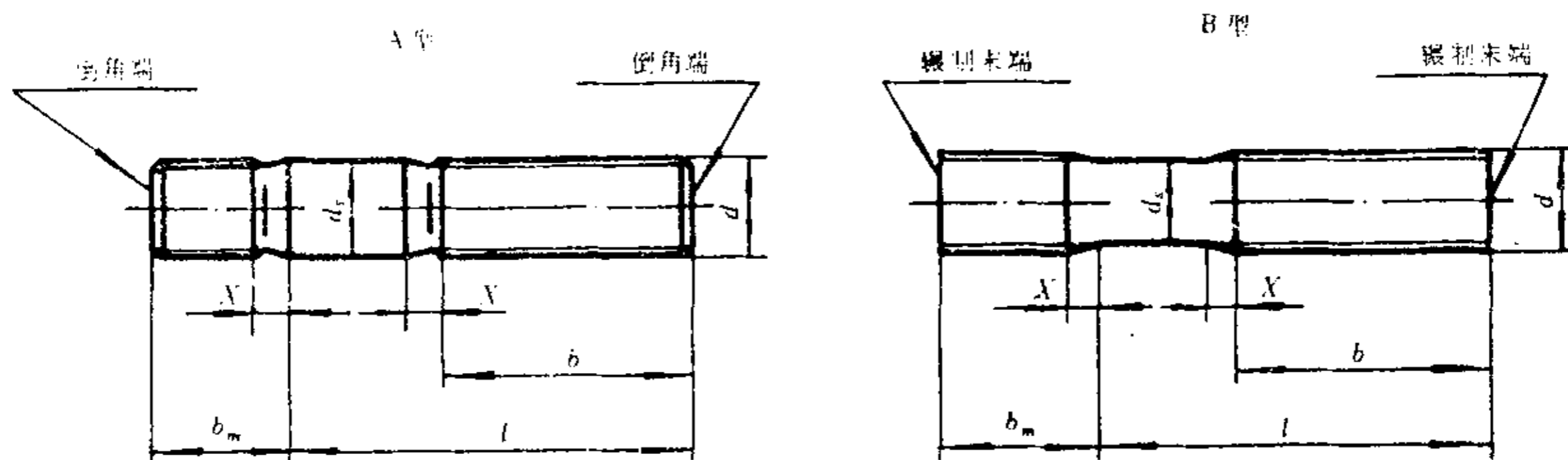
末端按GB 2规定： d_s \approx 螺纹中径（仅适用于B型）。
