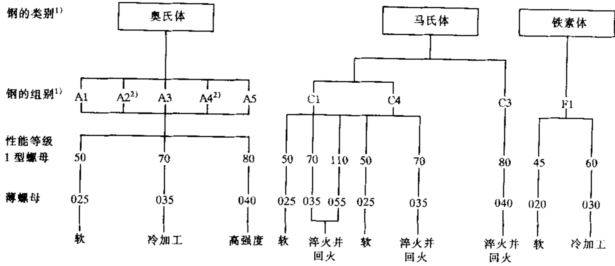
图1 螺母产品不锈钢组别和性能等级标记制度
