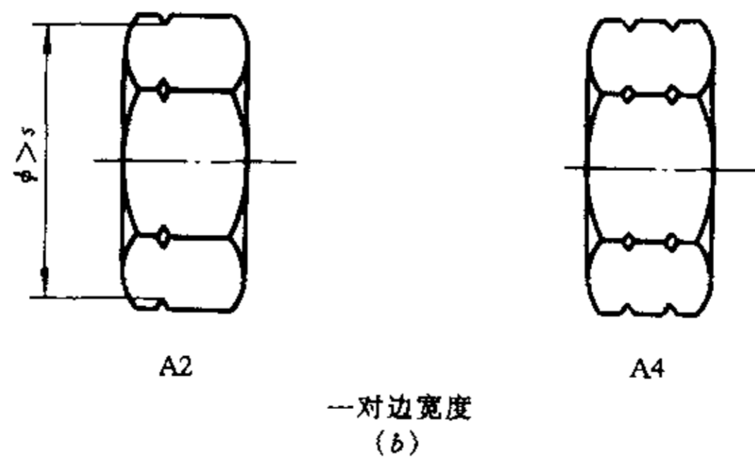
图2 螺母的标志
