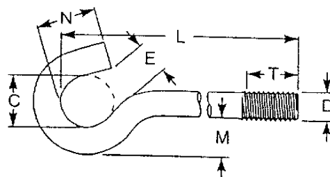
J-Bolt (DxLxCxExTxMxN)
