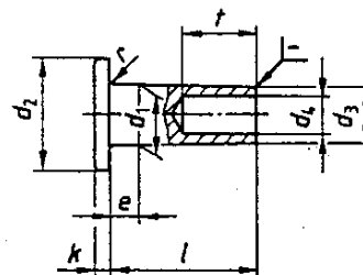
Type B, semitubular rivet
