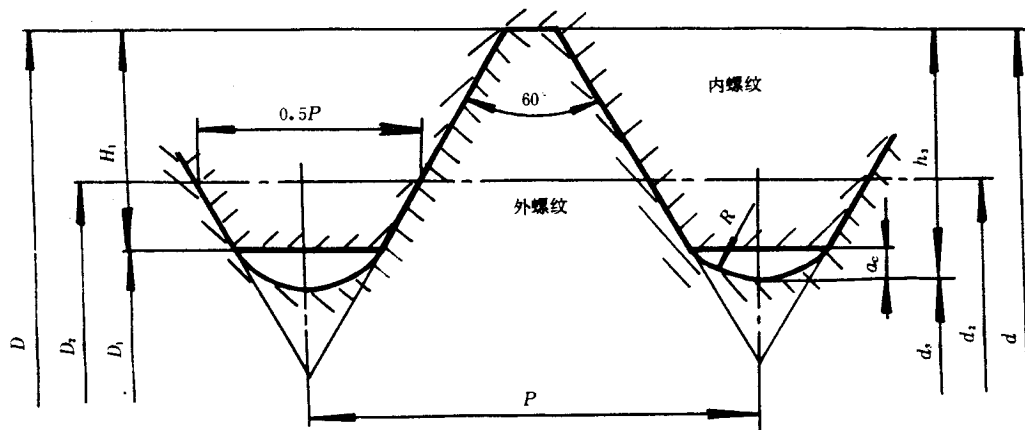
设计牙型的尺寸
