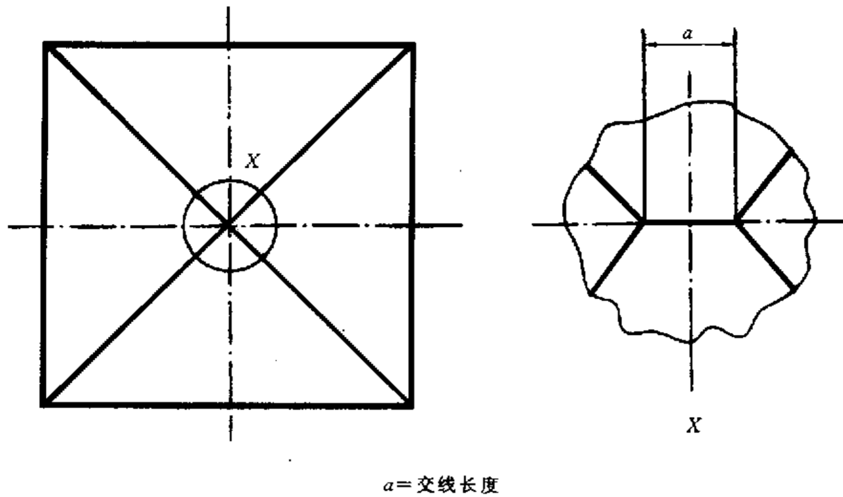
图 2 压头锥顶交线的示意图
