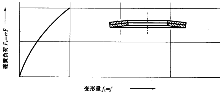
图 C.3 叠合组合碟簧
