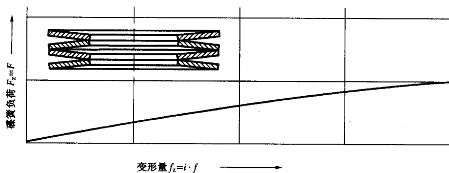
图 C.4 对合组合碟簧
