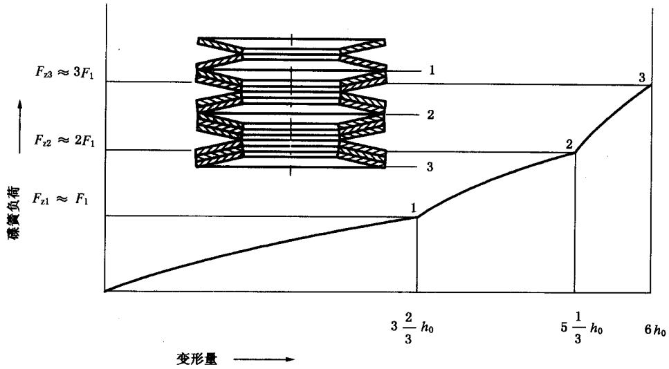
图 C.7 不同叠合片数的复合组合碟簧
