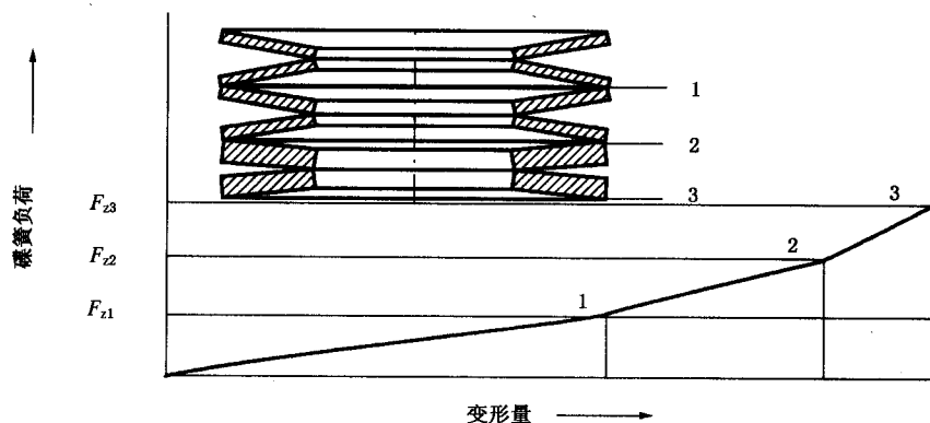
图 C.6 不同厚度的对合组合碟簧
