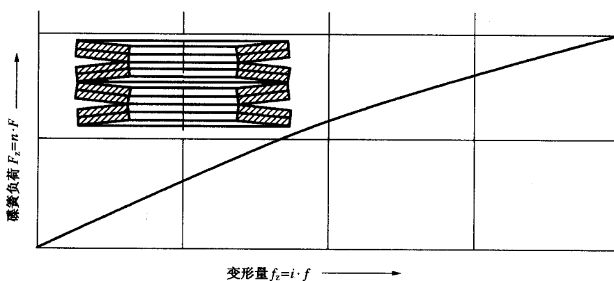
图 C.5 复合组合碟簧
