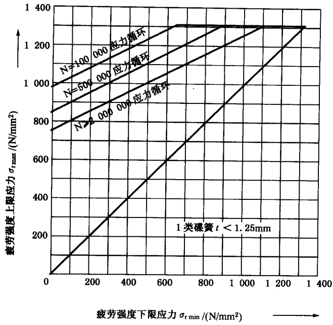
图 C.9 t < 1.25 mm 碟簧的疲劳强度曲线图
