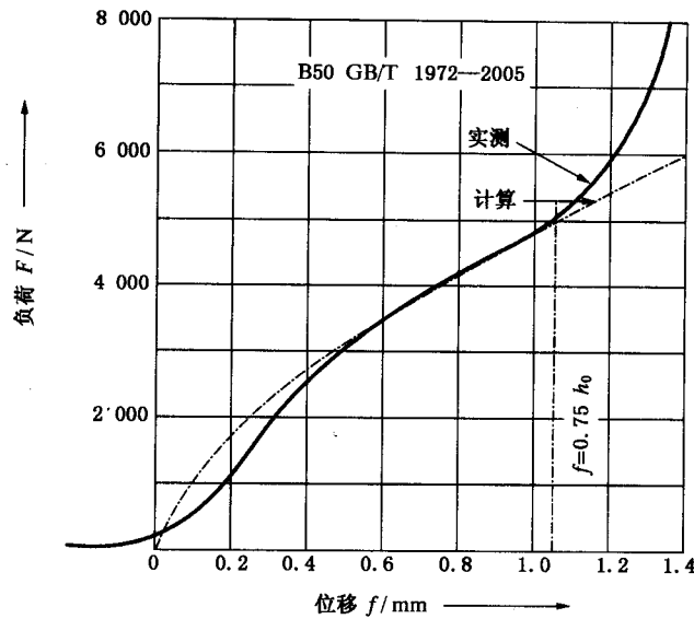
图 C.2 B50 碟簧计算和实测特性曲线
