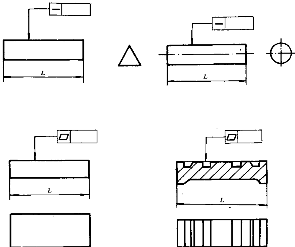
主参数 L 图例
