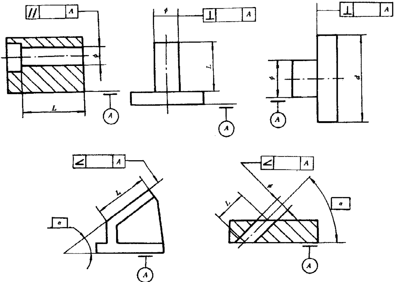
主参数 L, d(D) 图例
