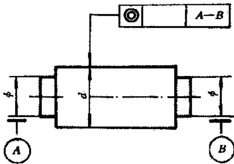
主参数 d(D), B, L 图例
