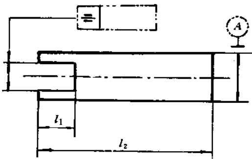
a) 基准: 较长要素 ( l_2 )
