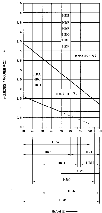
图 A.1 洛氏硬度(A、B、C、D、E、F、G、H 和 K 标尺)
