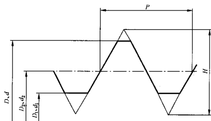
图 1 基本尺寸
