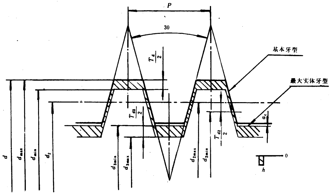
a. 大、中、小径的公差带位置为 h
